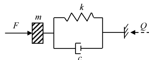
b) Kelvin-Voigt model
