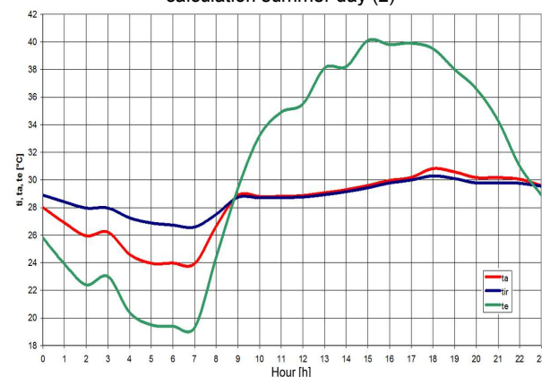
Fig. 25. Natural thermal regime – status b)
