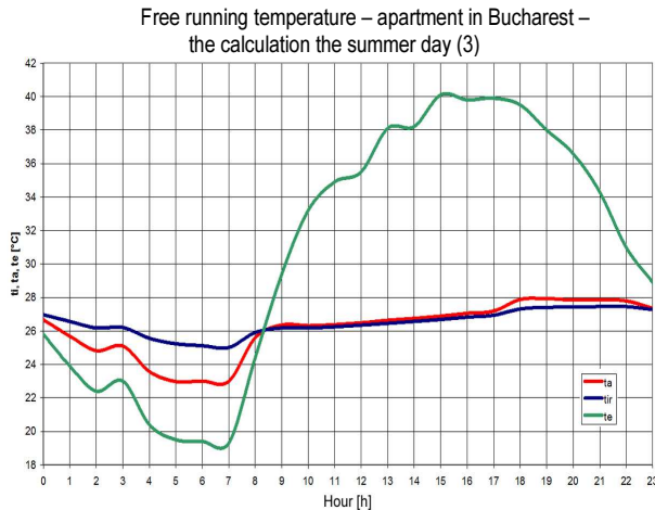
Fig. 27. Natural thermal regime – status c)
